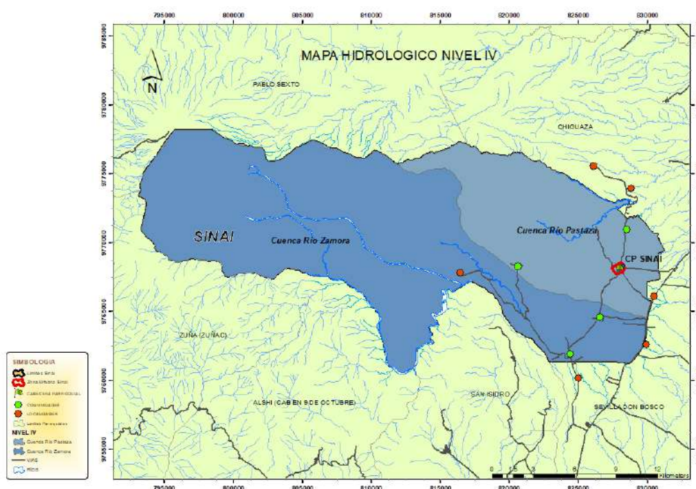
Ilustración 22: Mapa hidrológico nivel cuatro Fuente: MAATE 2017
