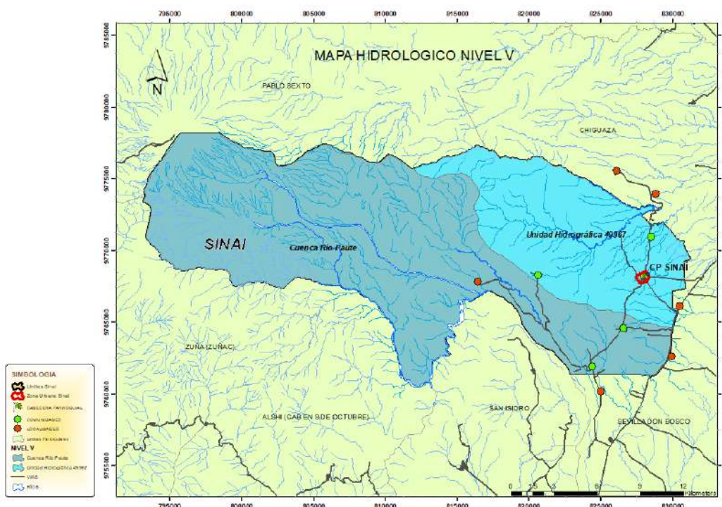
Fuente: MAATE 2017 Ilustración 23: Mapa hidrológico nivel cinco
