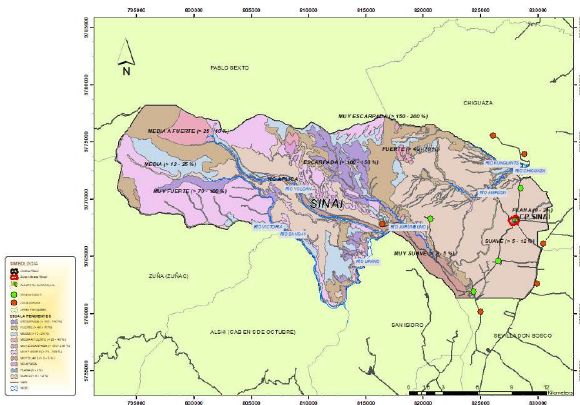
Ilustración 27: Mapa Pendientes Fuente: SIG TIERRAS 2016
