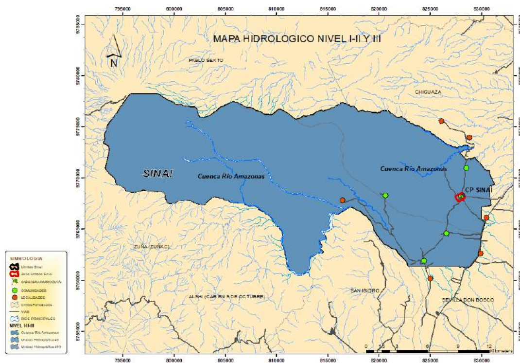
Ilustración 21: Mapa Hidrológico nivel III Fuente: MAATE 2017
