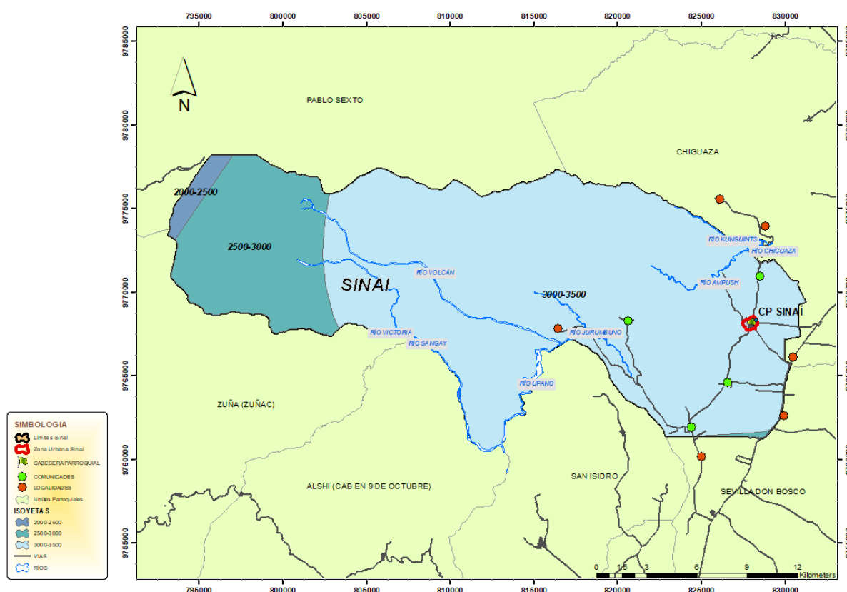
Ilustración 26: Mapa de precipitación Fuente: MAGAP 2011
