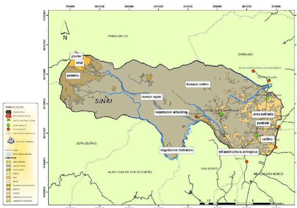
Ilustración 34: Mapa cobertura vegetal Fuente: MAE 2019
