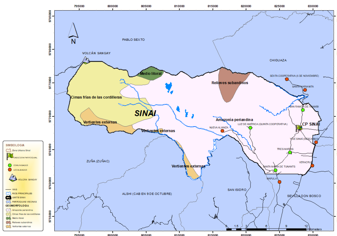
Ilustración 17: Geomorfología Fuente: Conali, 2023
