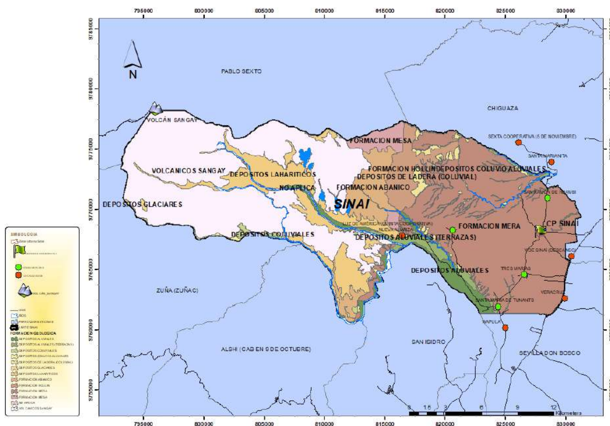
Ilustración 15: Geología Fuente: IERSE UDA 2019
